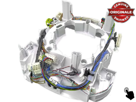
W-F32564 32564 Vorwerk ITA Modulo centrale completo di cablaggio per modello TM5 ENG Central module complete with wiring for TM5 model
