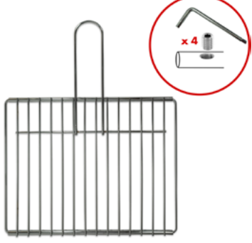
WY321 Universale ITA Griglia barbecue cromata estensibile misure M 380x310 mm allungabile 640x310 mm con vite a scomparsa e chiavetta di montaggio ENG Barbecue Grille CHROMED "M" 380X310 cm extensible 640X310 cm With recessed scre W and mounting key
