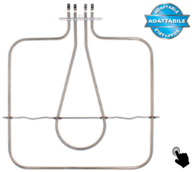
WA200 41000114 - 41020672 Candy ITA Resistenza per forno doppia 1050+450 W 230v/98v adattabile - 2371 ENG Oven heating element 1050+450 W 230V/98V adaptable
