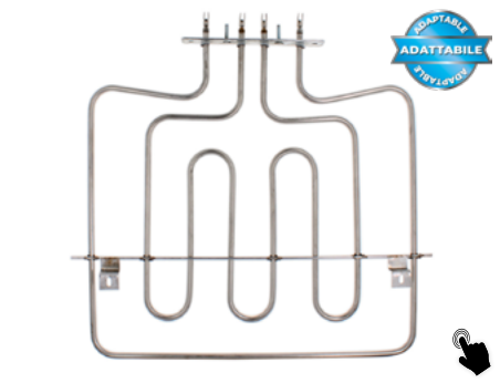
WA204 3570337018 - 50208855002 Electrolux ITA Resistenza per forno doppia 1200/1800 W 230v adattabile ENG Oven heating element 1200/1800 W 230V adaptable
